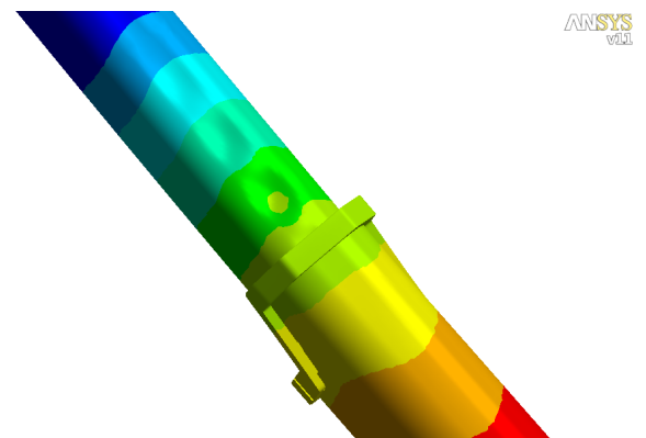
Verschiebungen in Profilhochachse aus Traglastberechnung (überhöhte Darstellung)
