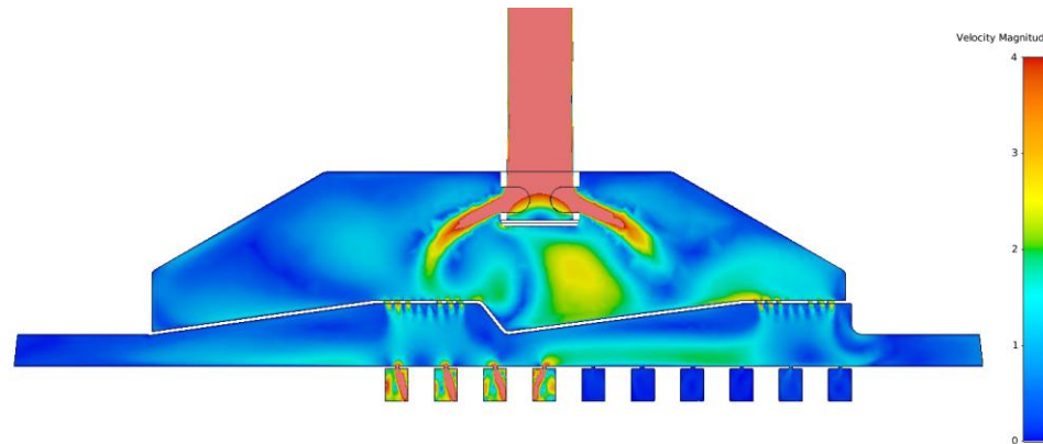
Dampfblaskasten in einer Papiermaschine
